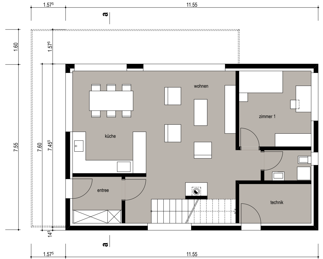
grundriss dachgeschoss haus A 1:100
