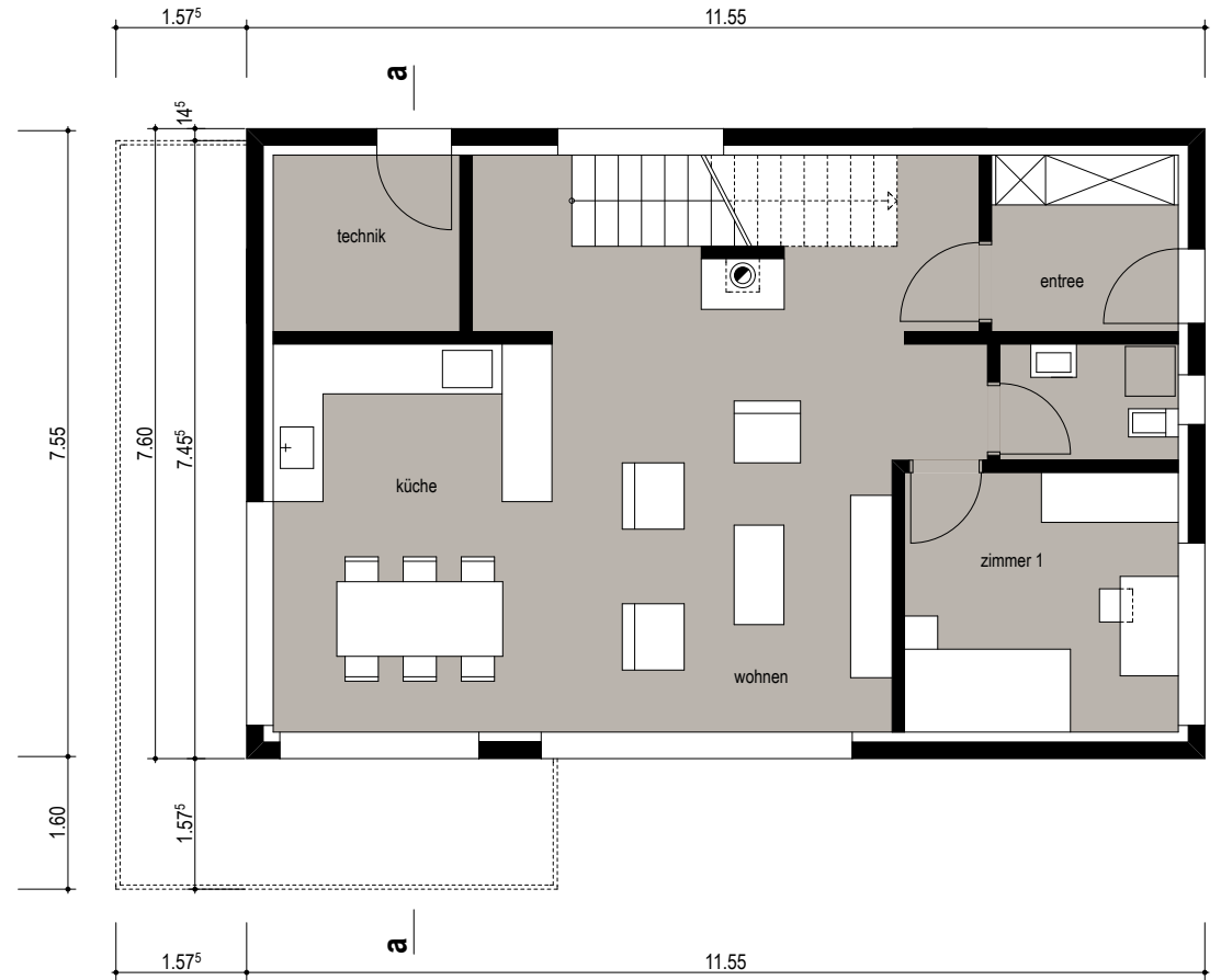
grundriss dachgeschoss haus B 1:100
