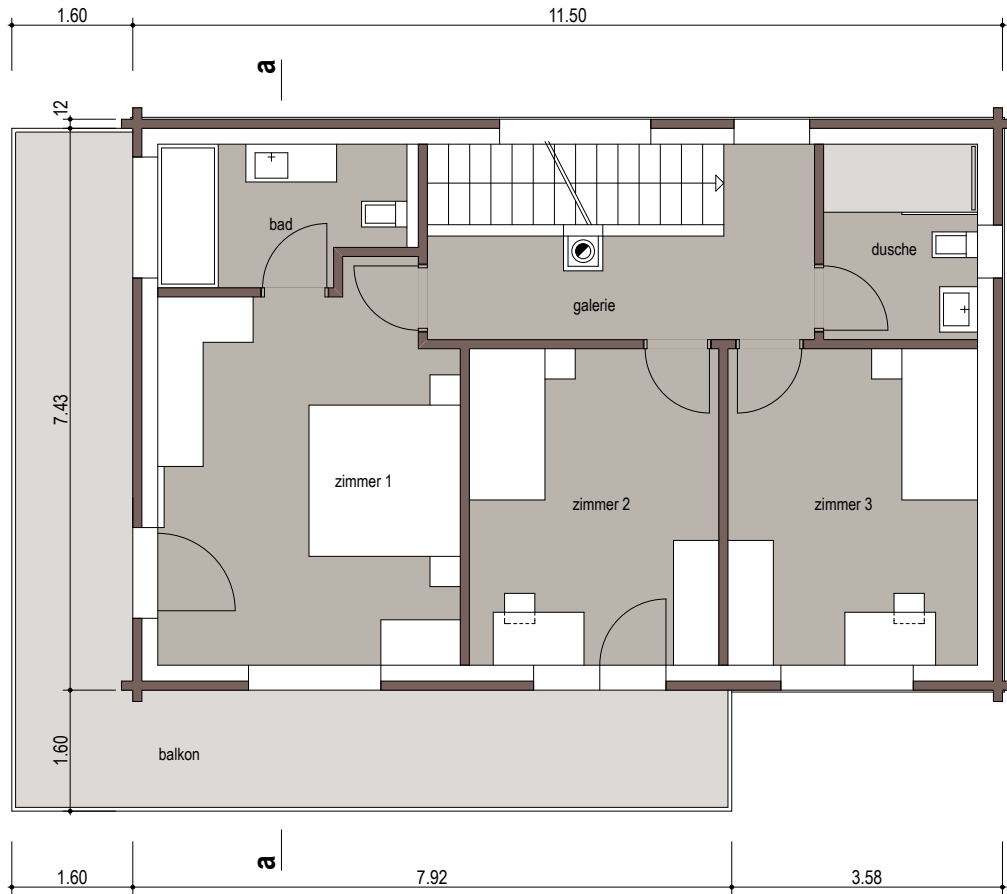
grundriss erdgeschoss haus B 1:100
