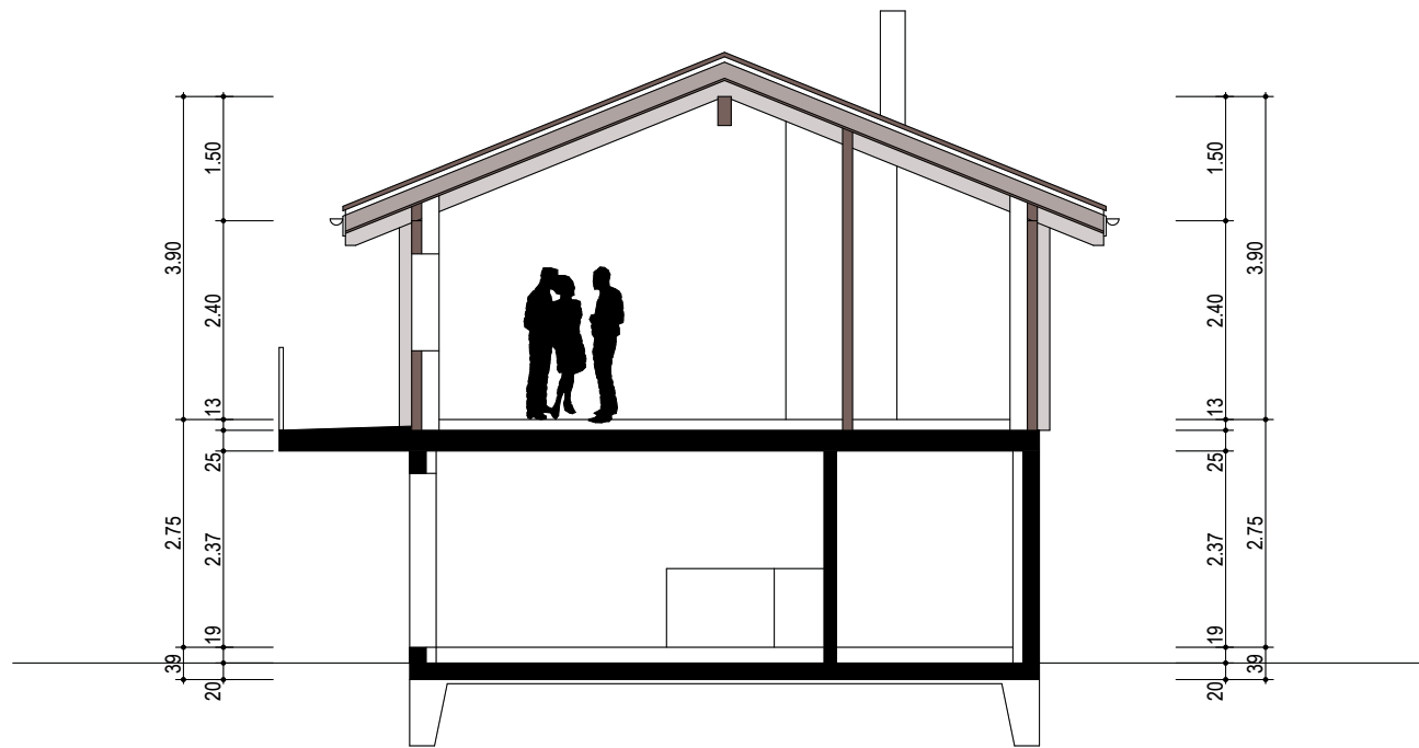
schnitt a--a 1:100
